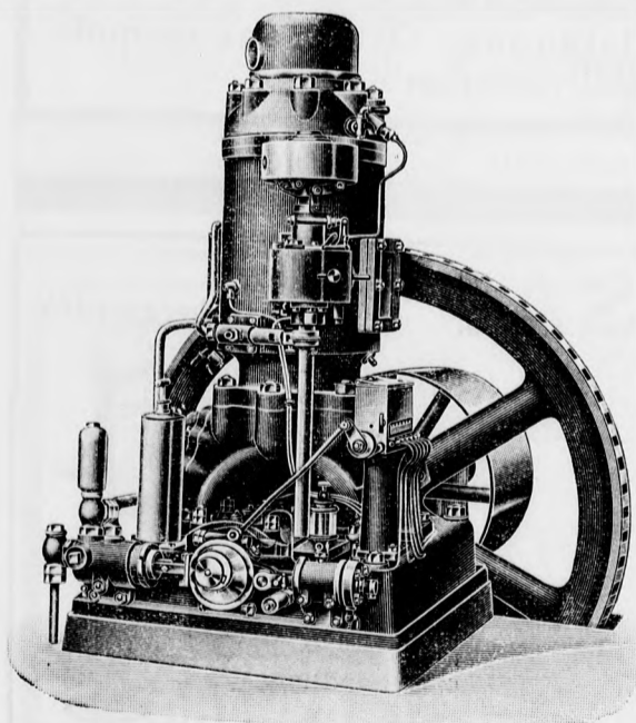
35 HP 2 cylinderes kivitel.
