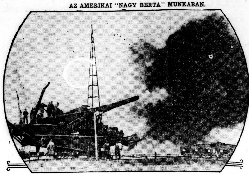
Amerikának legnagyobb ágyúja gyakorlat közben. A jövő háborújának egyik legnagyobb és legmesszebb hordó ágyúja. Most próbálják ki, és azt mondják, hogy megfelel a célnak, a melyre szánták.
