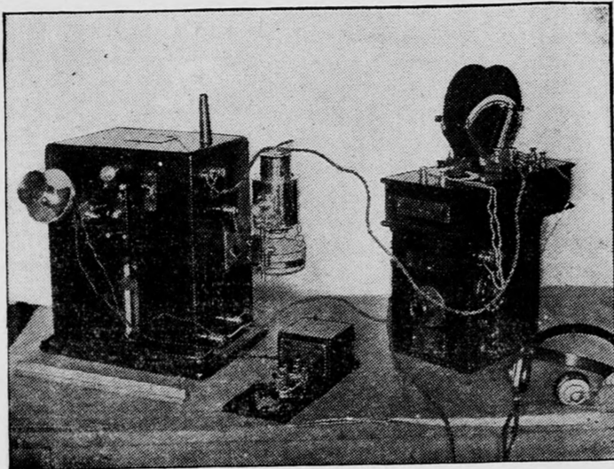
Drótnélküli telefon felszerelése.
