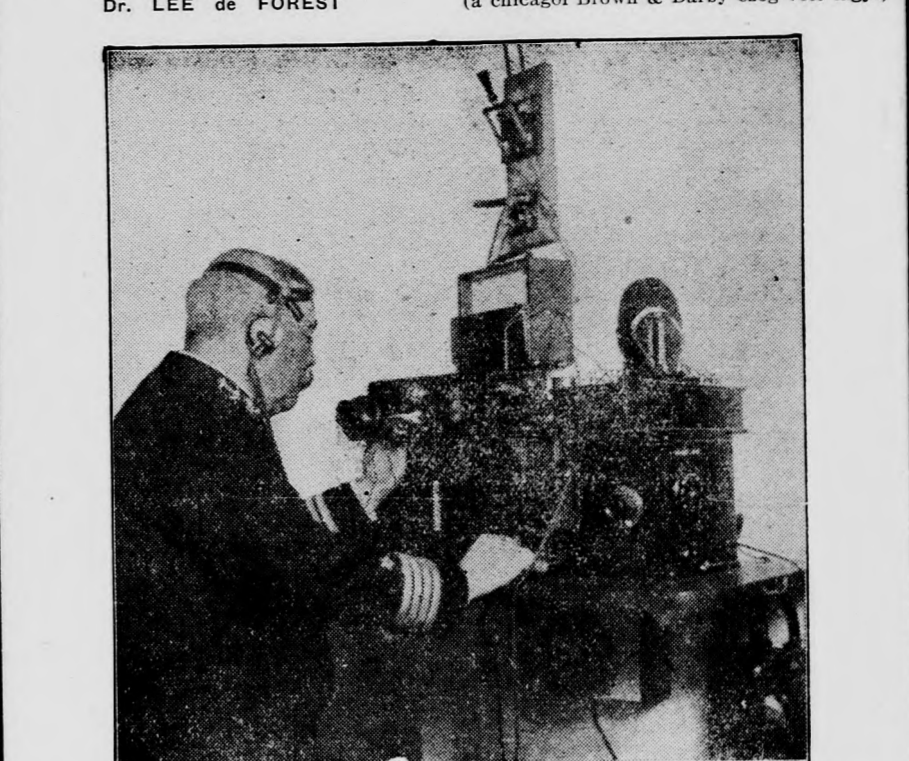
Ingersoll kapitány, „Bob” Evans tengernagy vezérkari főnöke, amint a tengernagy zászlóshajóján, az Egyesült Államok „Conncticut” nevű hadihajóján a „Radio Telephone” (De Forest drótnélküli telefonját) használja. A „Conncticut” az első állomás a telefon-összeköttetésre a nyílt tengeren két egymástól eltávolított hajó között. Az Egyesült Államoknak pacific-hajóira, mely több mint 30 hadihajóval, cirkálóikkal, torpedórombolókkal áll, fel van szelve a drótnélküli teleffonnal.
