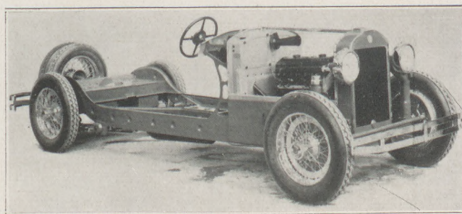
Lancia-Dilambda
