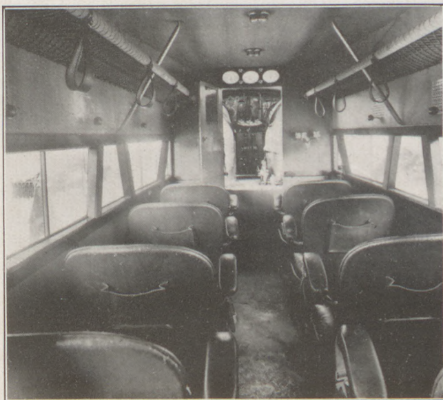
A »Cidna«-gép belseje
