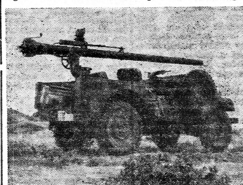
Az amerikai gyártmányú 106-os páncéltörő ágyú
