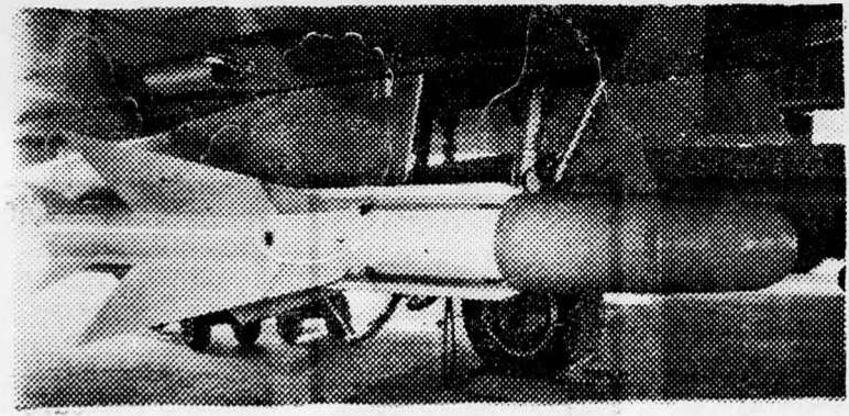
A „Matra 530-R” közelről, a Mirage repülőgépre szerelve, kilőésre kész állapotban
