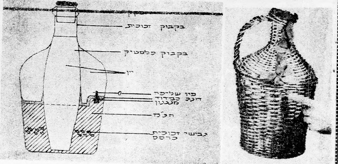
A robbanó borospalack belső szerkezete a robbanó anyaggal, gyújtószerkezettel és üvegszálakkal
